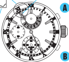
Anno (numero di anni trascorsi dall'ultimo anno bisestile)
